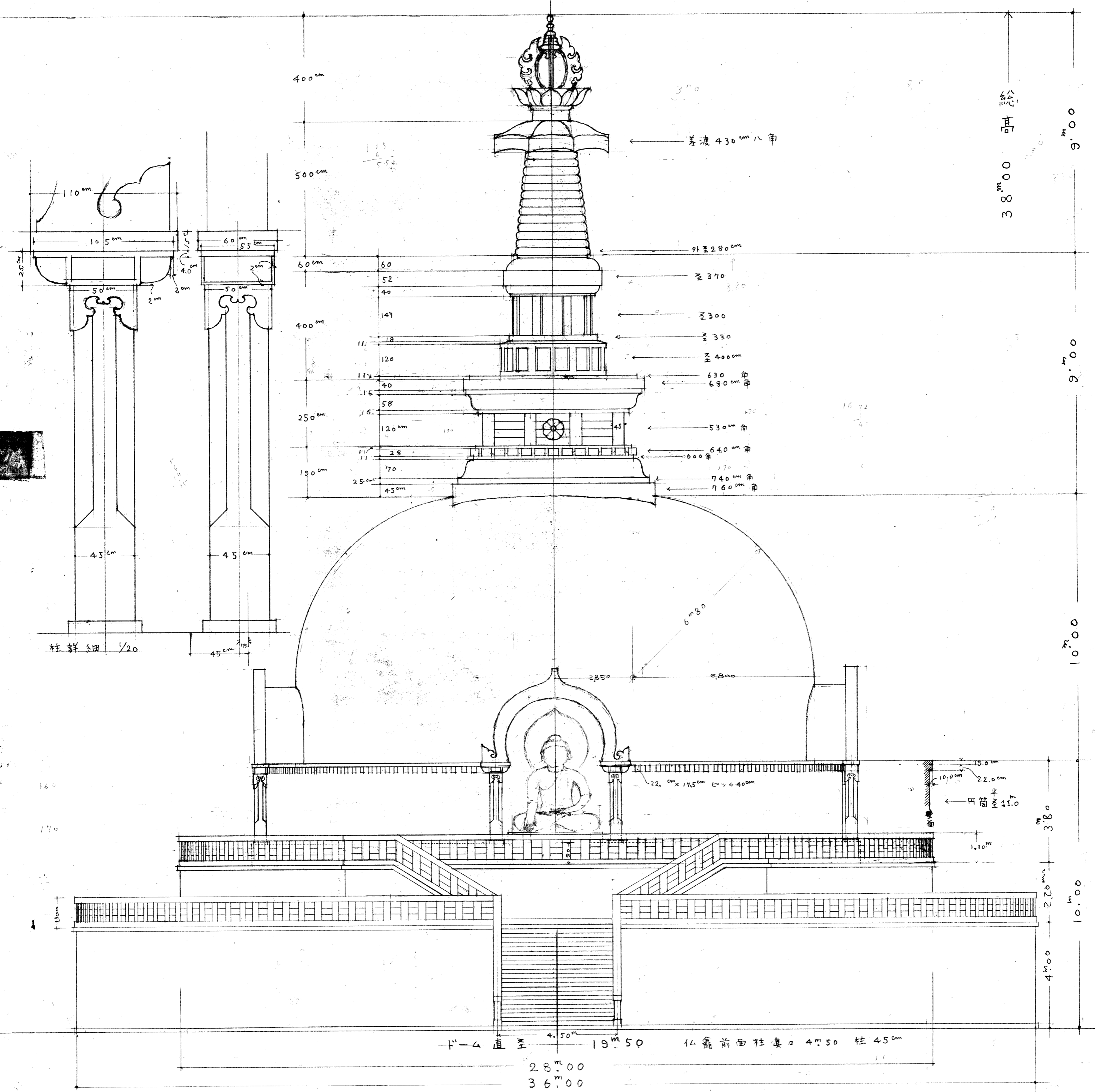
牛津仏舎利塔正立面図 S = 1:100. 昭.51.8.3 圖
